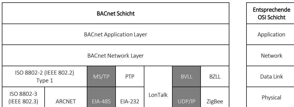
Figure 12 : Architecture BACnet simplifiée (selon [1])
